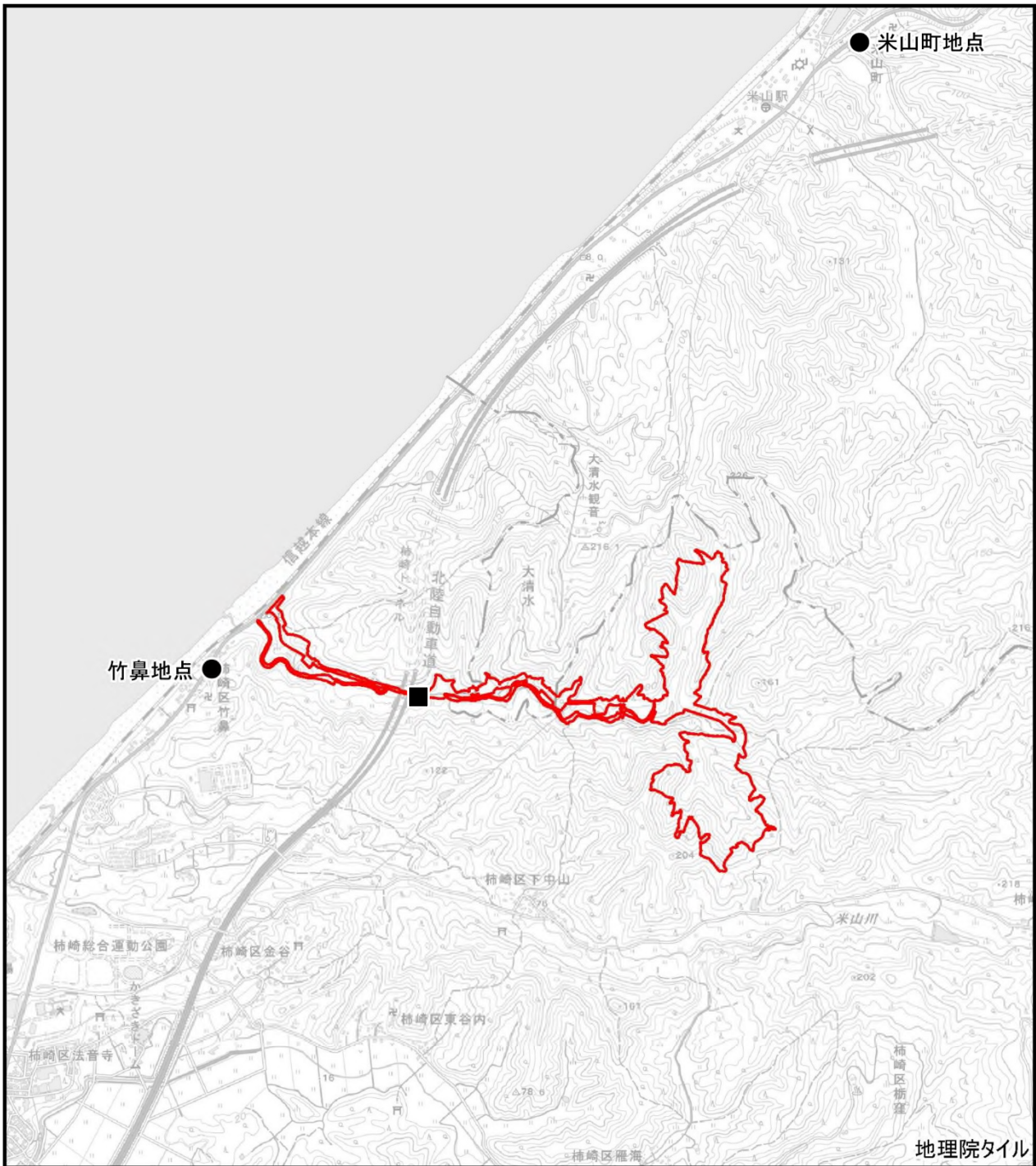
図 5.2-1 窒素酸化物、浮遊粒子状物質等の調査地点位置図
