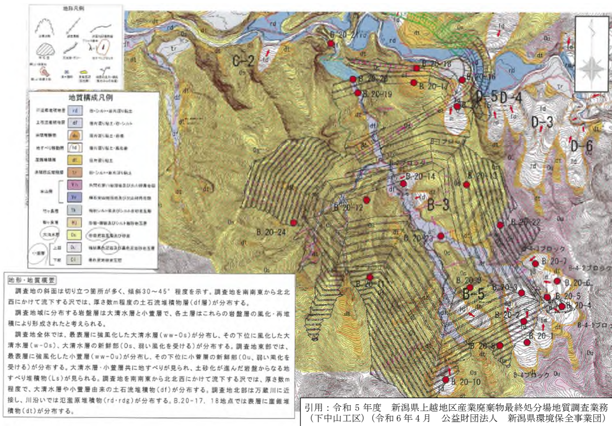
図 6.1-44 地質平面図（下中山地区埋立地）
