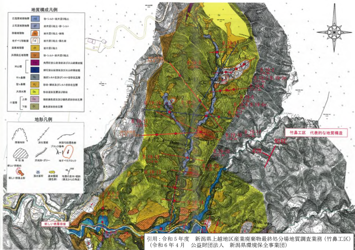
図 6.1-43 地質平面図（竹鼻地区埋立地）
