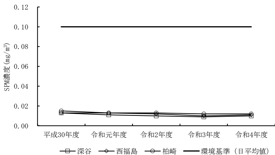
図 6.1-4 浮遊粒子状物質（年平均値）の経年変化
