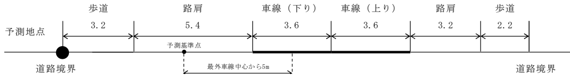
図 6.1-51 (2) 道路交通振動 予測断面図 (米山地点)
