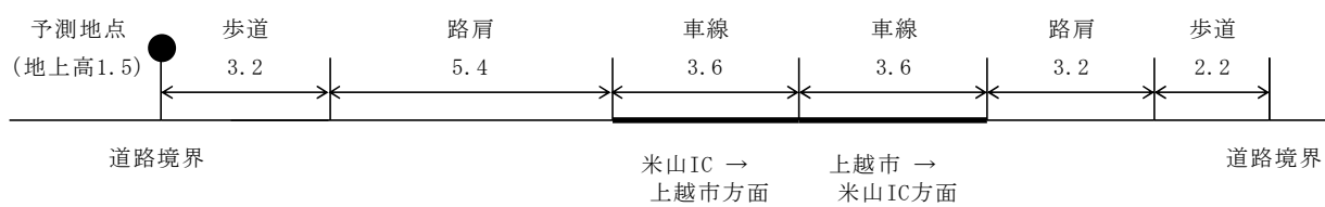
図 6.1-18 (2) 米山町地点の道路構造
