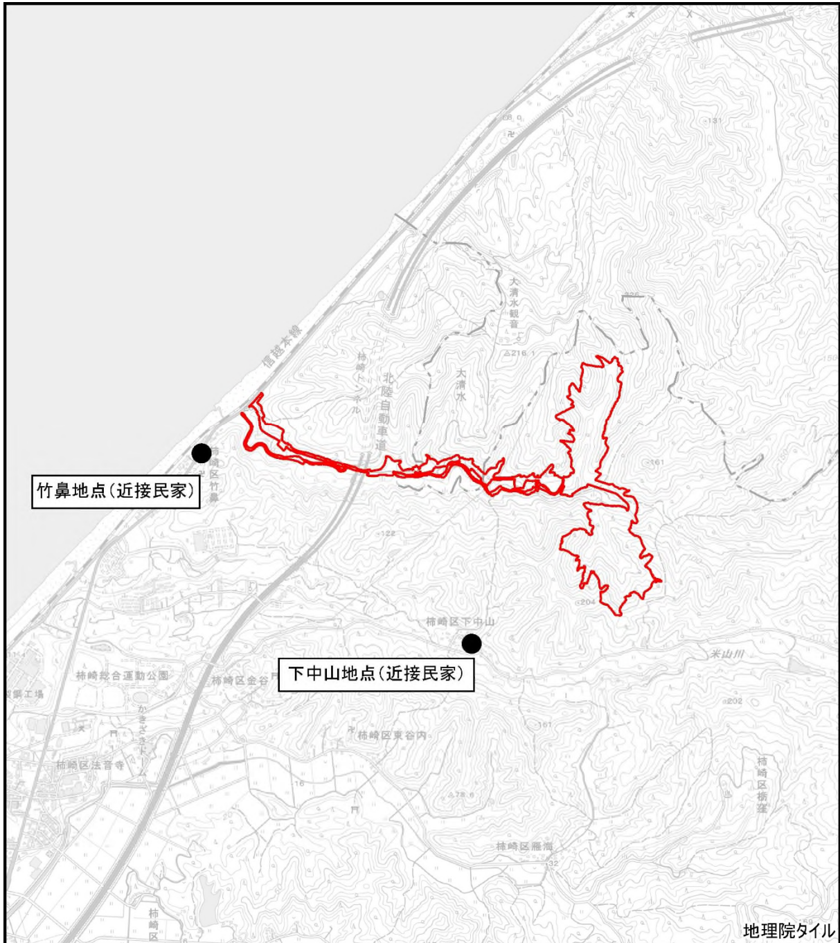
図 6.1-46 建設機械の稼働（工事用道路）に伴う振動 予測地点位置図
