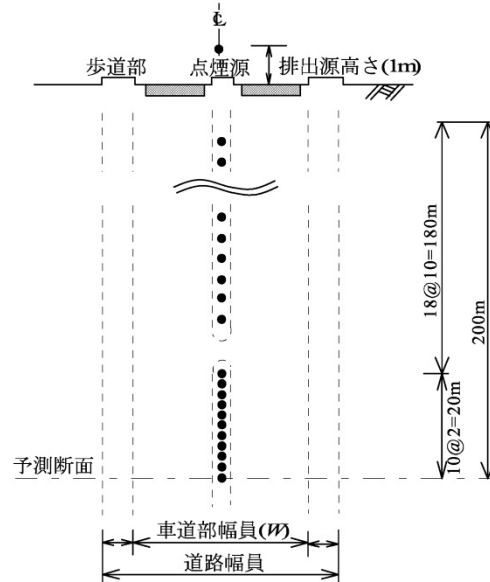
図 6.1-19 点煙源の配置
